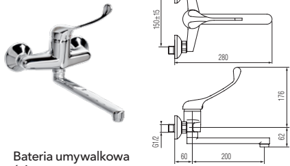
Bateria umywalkowa ścienna
