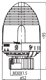
Kod zawór VECTOR X 4440000 zawór IRIS przyłłącze M30x1,5 (typ Heimeier) Danfoss z przyłączem RA - w przypadku grzejników z wkładką typu DAN-FOSS należy zastosować adapter - 4445110
