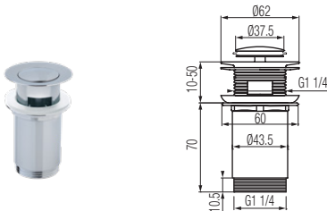
Automatyczny korek spustowy
