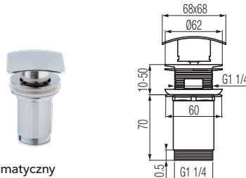
Automatyczny korek spustowy
