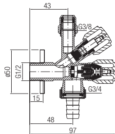
Kod Wymiary P nom. / max temp. 1482100 1/2"-3/8"-3/4" PN 10 / 80°C
