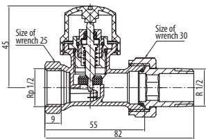
Kod Kolor Wymiar D d L Lk I H S S1 P nom. 4411010 NIKLOWANY 3/8" Rp3/8 R3/8 75 50 9 41,5 22 27 PN 10 4412010 NIKLOWANY 1/2" Rp1/2 R1/2 82 55 10 41,5 27 30 PN 10 4413010 NIKLOWANY 3/4" Rp3/4 R3/4 98 65 12 43 32 37 PN 10 4412090 BIAŁY 1/2" Rp1/2 R1/2 82 55 10 41,5 27 30 PN 10
