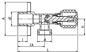
Kod Wymiary P nom. / max temp. Rozmiar A L I Lk d d1 h 1484050 1/2"-3/8" 50 88 14 39,5 G3/8 G1/2 24 PN 10 / 90°C 1484060 1/2"-1/2" 50 88 14 39,5 G1/2 G1/2 24 PN 10 / 90°C 1484070 1/2"-3/4" 50 88 14 39,5 G3/4 G1/2 24 PN 10 / 90°C
