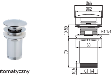
Automatyczny korek spustowy
