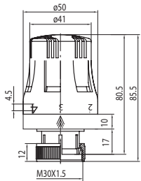
Kod zawór VECTOR 4445050 zawór IRIS X przyłłącze M30x1,5 (typ Heimeier) X Danfoss z przyłączem RA - w przypadku grzejników z wkładką typu DAN-FOSS należy zastosować adapter - 4445110
