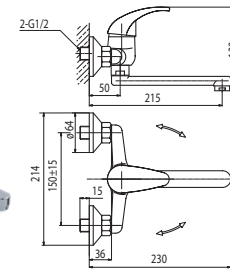
Bateria umywalkowa ścienna
