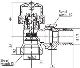
Kod Kolor Wymiar Wymiary P nom. D d L Lk I H h S S1 4512010 NIKLOWANY 1/2" Rp1/2 R1/2 53 26 10 41,5 23 27 30 PN 10 4513010 NIKLOWANY 3/4" Rp3/4 R3/4 63 30 12 43 26 32 37 PN 10 4512090 BIAŁY 1/2" Rp1/2 R1/2 53 26 10 41,5 23 27 30 PN 10
