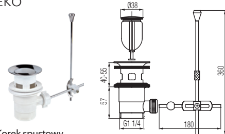
Korek spustowy z tworzywa z ciągnem
