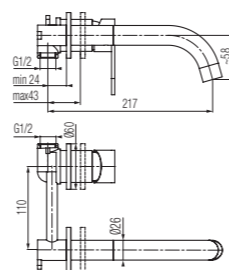
Bateria umywalkowa podtynkowa
