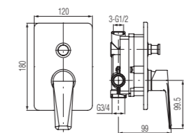
Bateria wannowo-natryskowa podtynkowa
