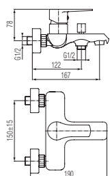
Bateria wannowa ścienna
