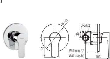
Bateria natryskowa podtynkowa
