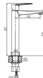
Bateria umywalkowa wysoka
