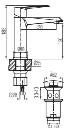
Bateria umywalkowa wysoka
