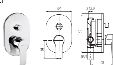
Bateria natryskowa podtynkowa
