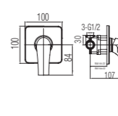
Bateria natryskowa podtynkowa
