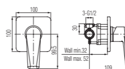
Bateria natryskowa podtynkowa
