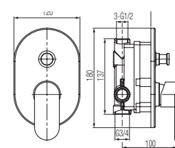
Bateria wannowo-natryskowa podtynkowa
