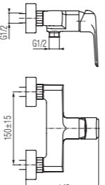
Bateria natryskowa ścienna
