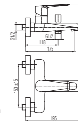
Bateria wannowa ścienna
