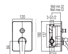
Bateria podtynkowa 2-funkcyjna
