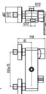
Bateria natryskowa 2-funkc.
