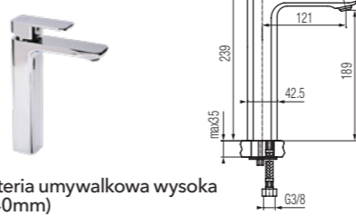
Bateria umywalkowa wysoka (270mm)
