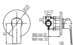
Bateria natryskowa podtynkowa
